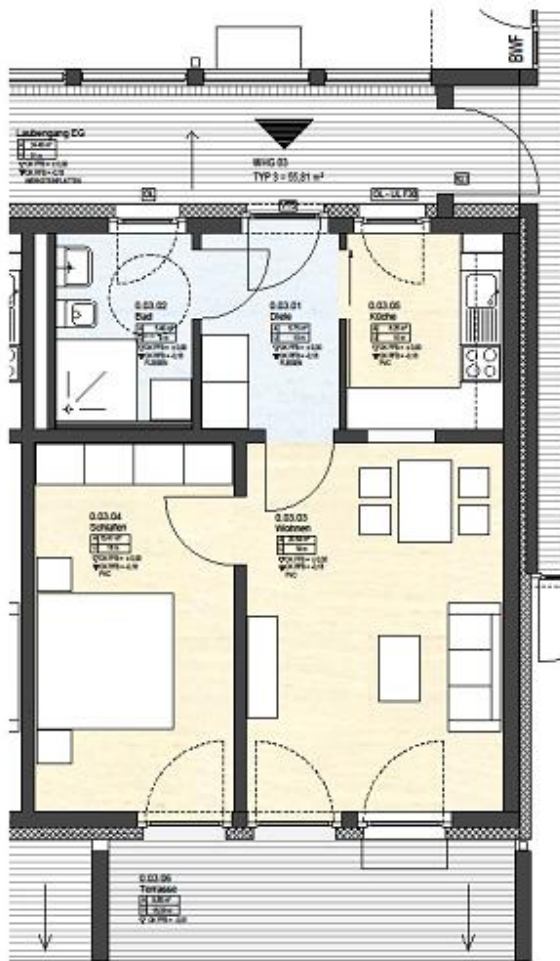
Wohnungstyp III
